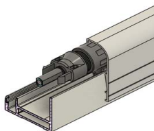
Horizontales Kabelmanagement im PV-Modul mittels Kabelleiste.
