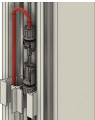
Vertikales Kabelmanagement im Solar-Pfosten.
