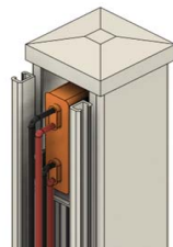
Optionale Aufnahme von Leistungsoptimierern versteckt im Solar-Pfosten.
